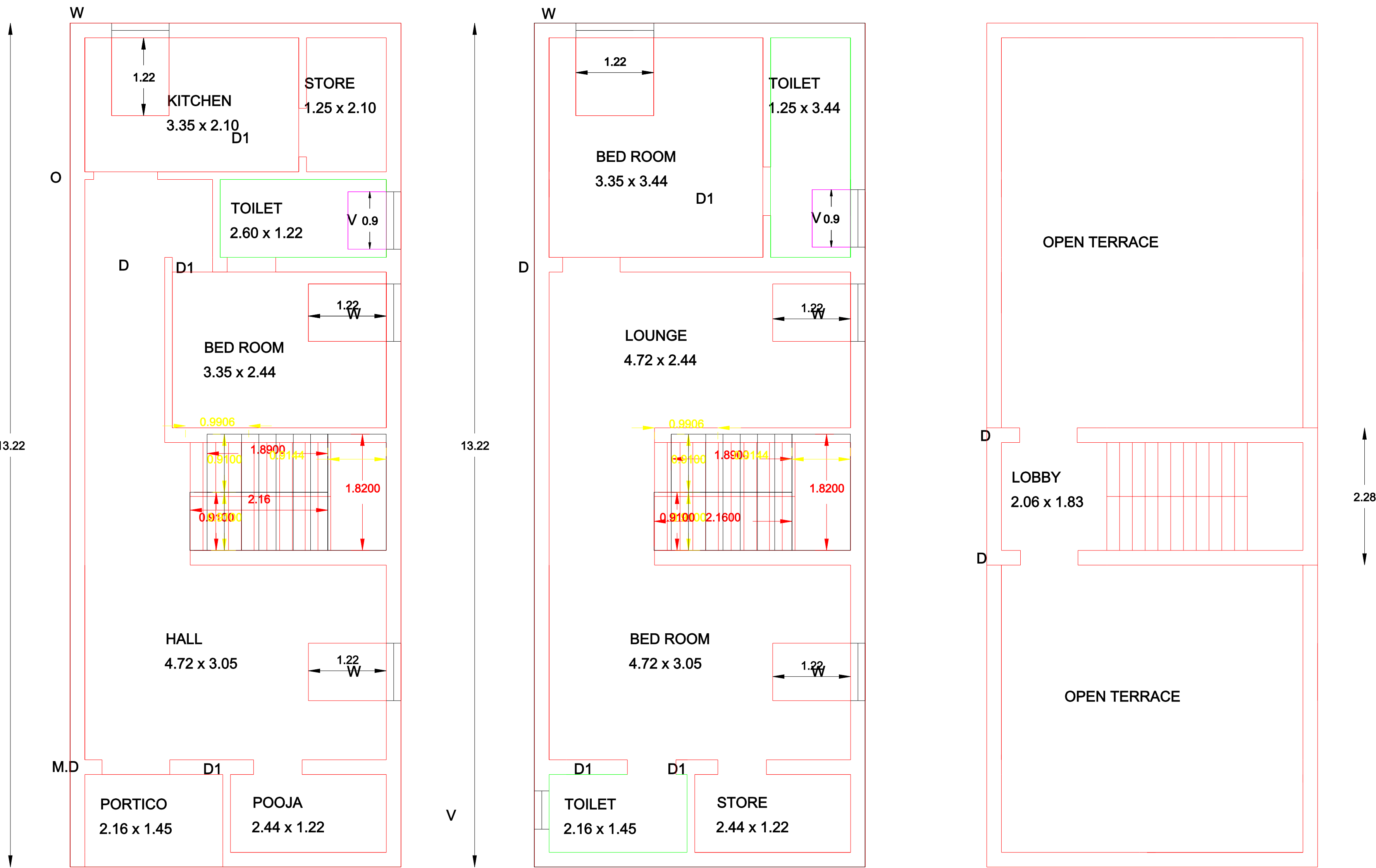
DOOR PLAN
