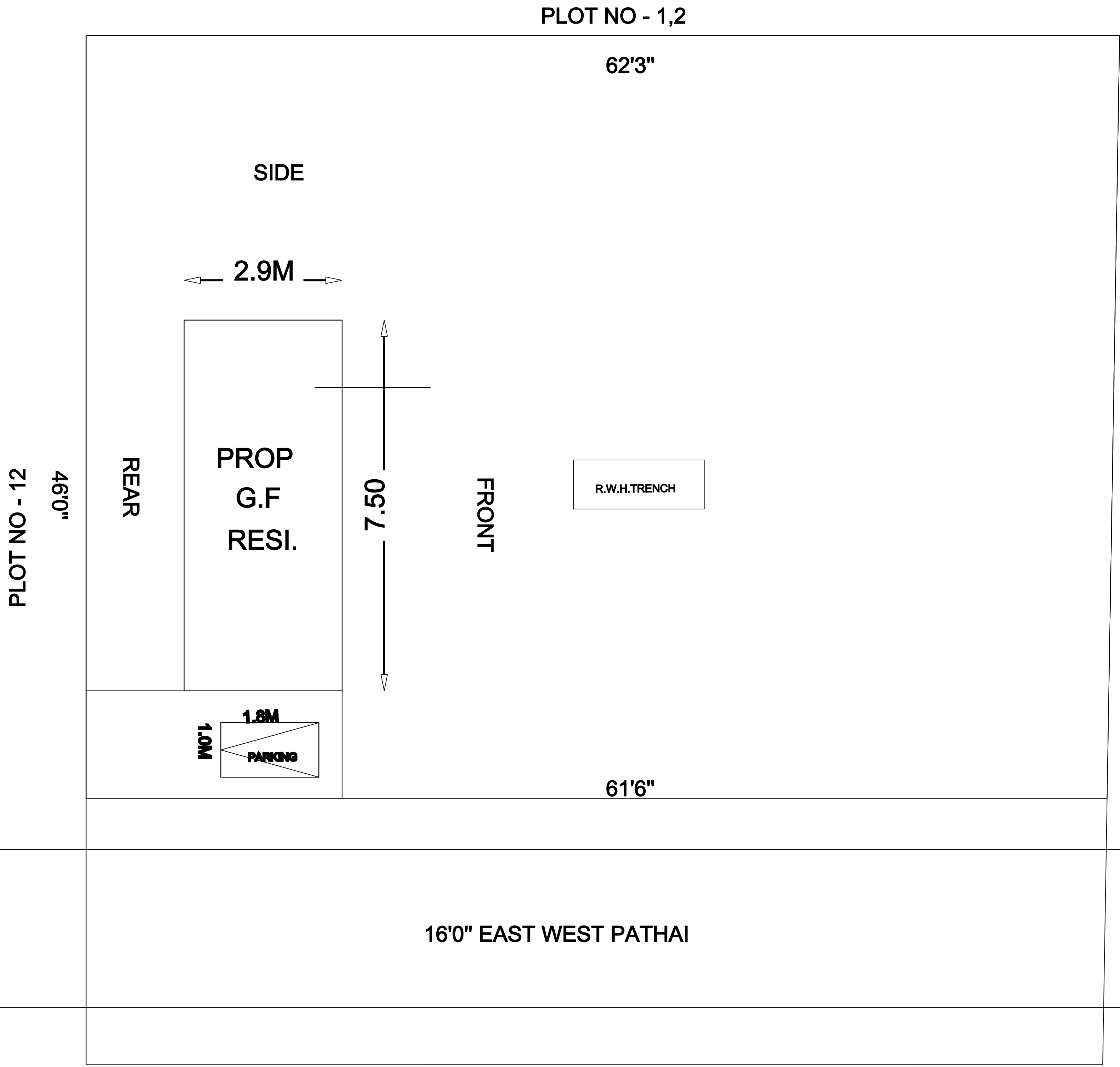
SITE PLAN, SCLAE- 1:100
