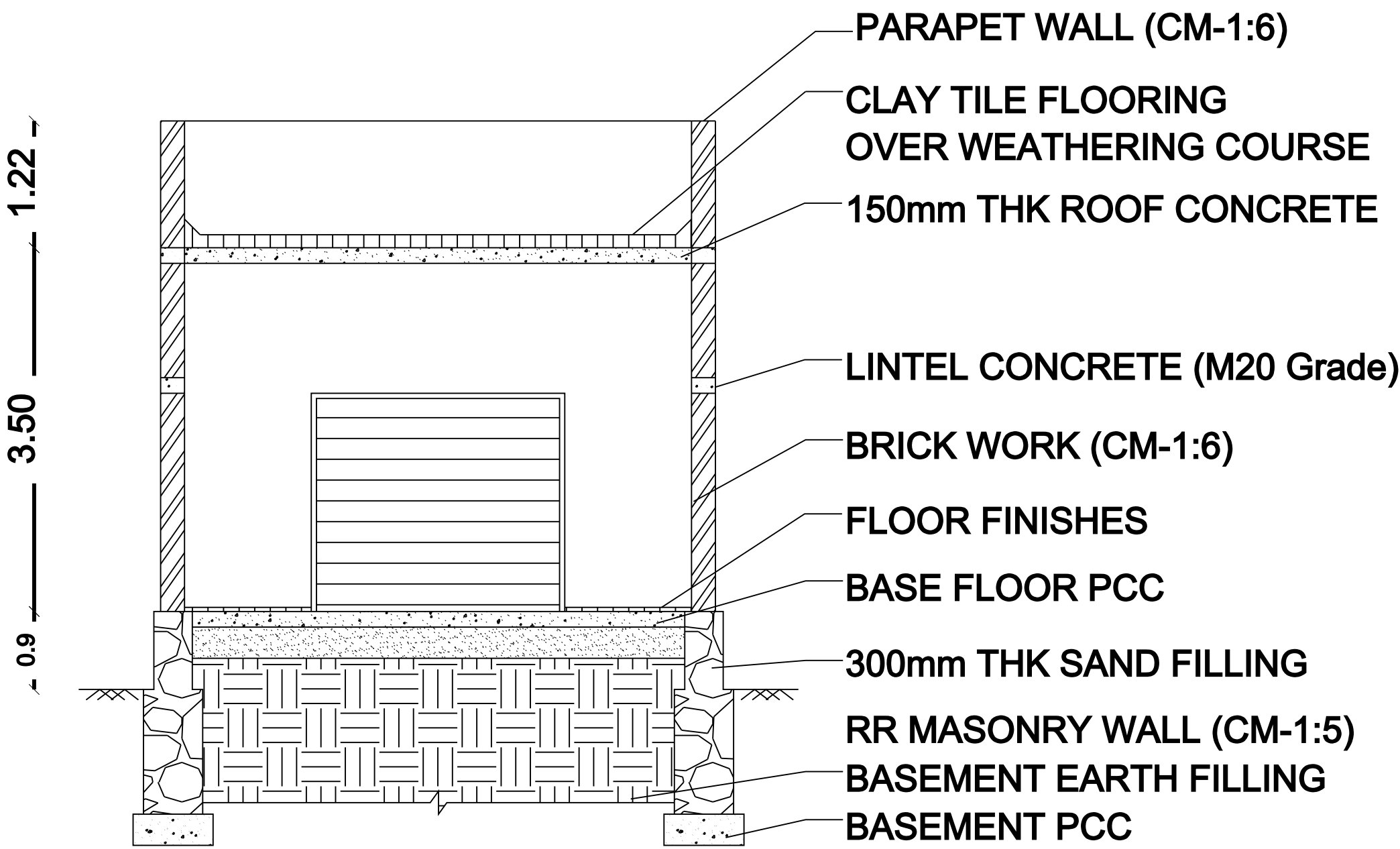
SECTION A-A
