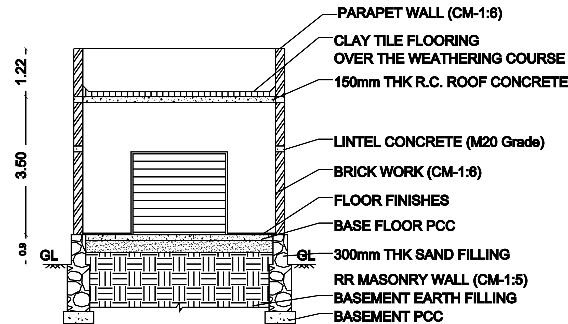
SECTION A-A
