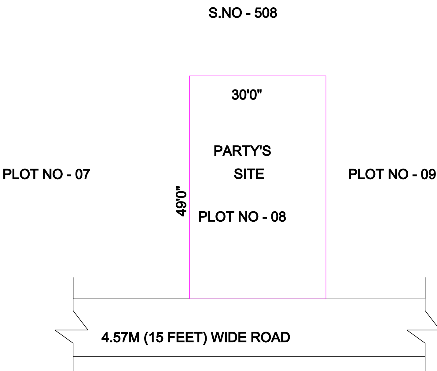
SITE PLAN SCALE 1:4
