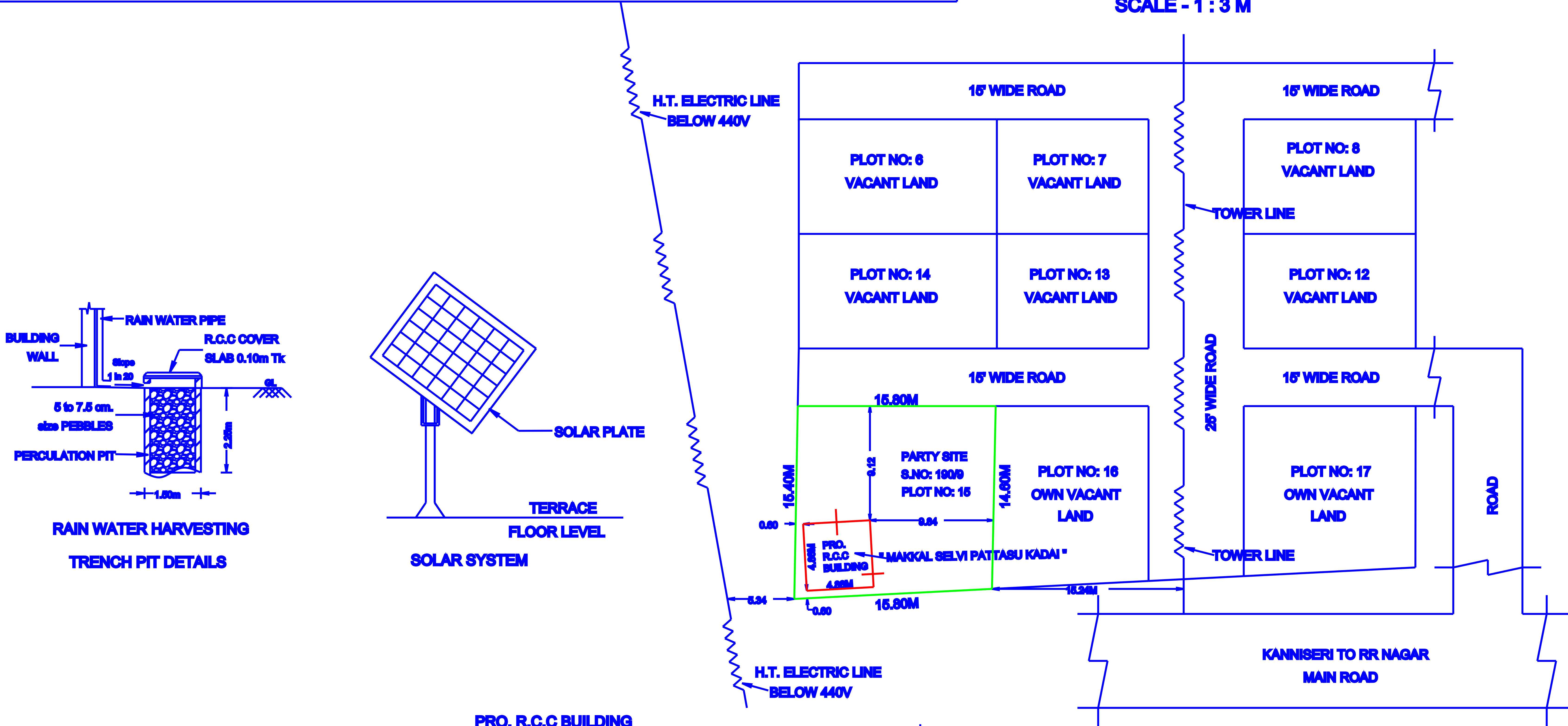
SITE PLAN SCALE - 1 : 3 M
