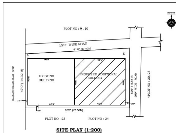
SITE PLAN (1:200)
