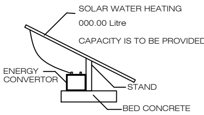
LONGITUDINAL SECTION
