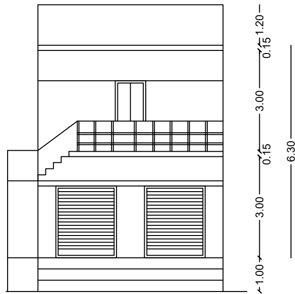
ELEVATION
