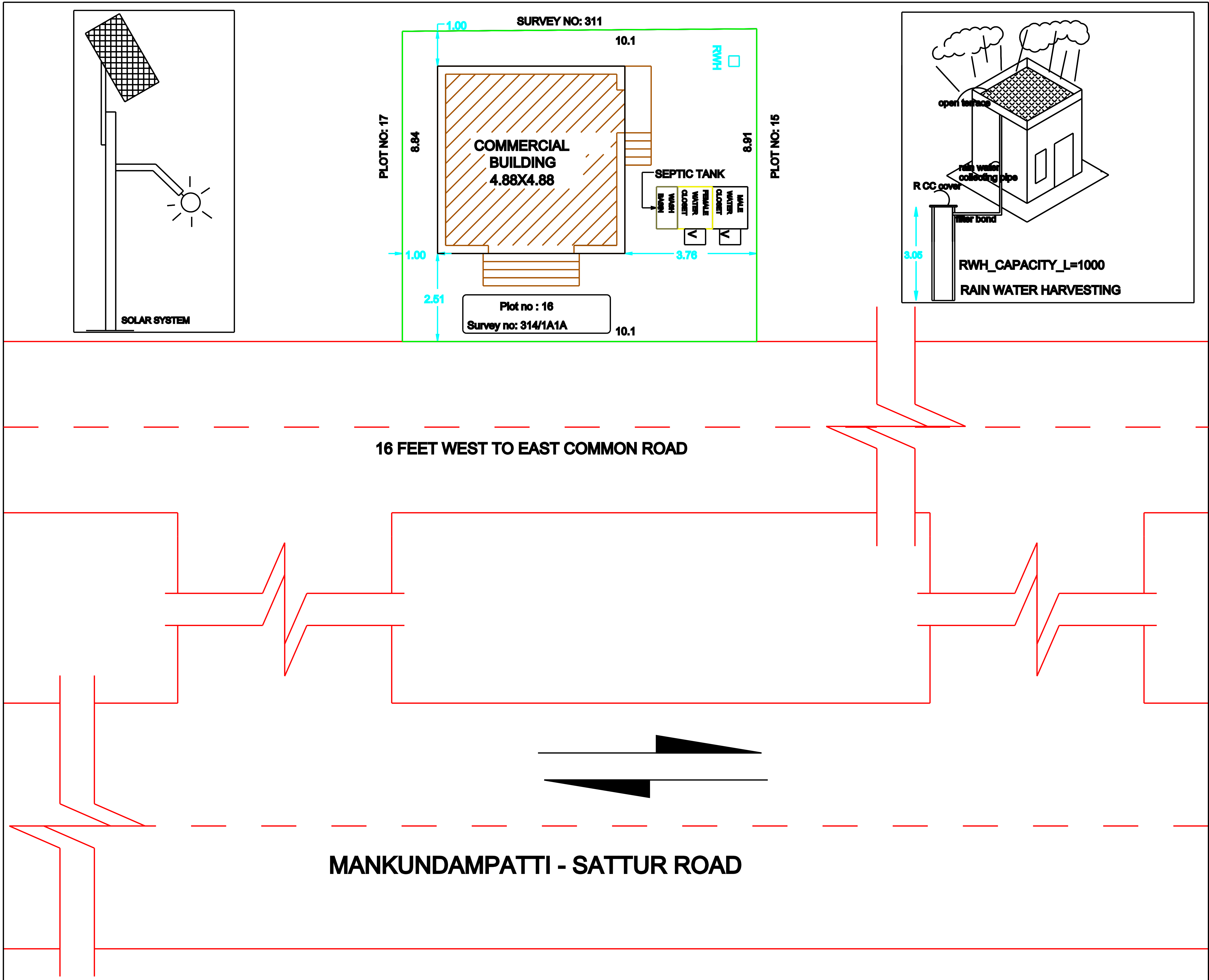
SITE PLAN SCALE 1:100
