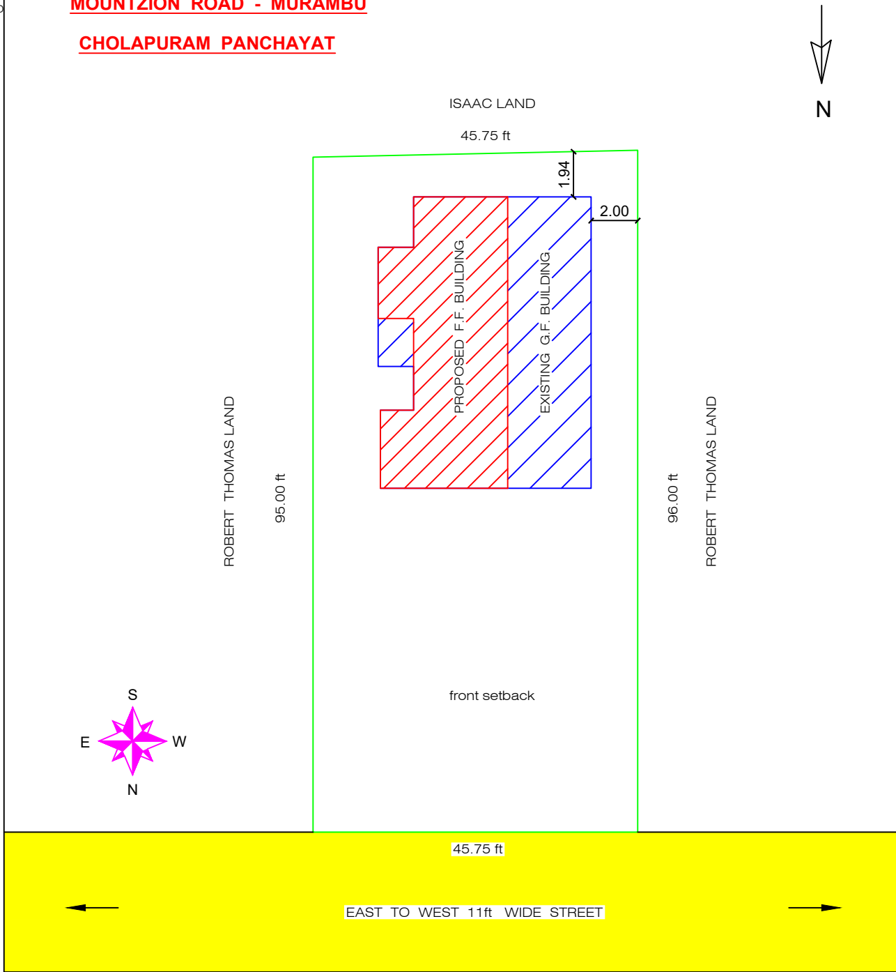
SITE PLAN SCALE : 1:50.
