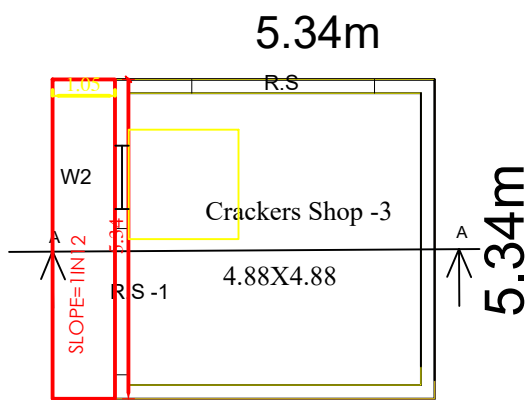
PRO. PLAN
