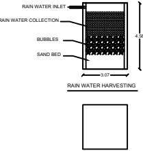
PLAN R.W.H
