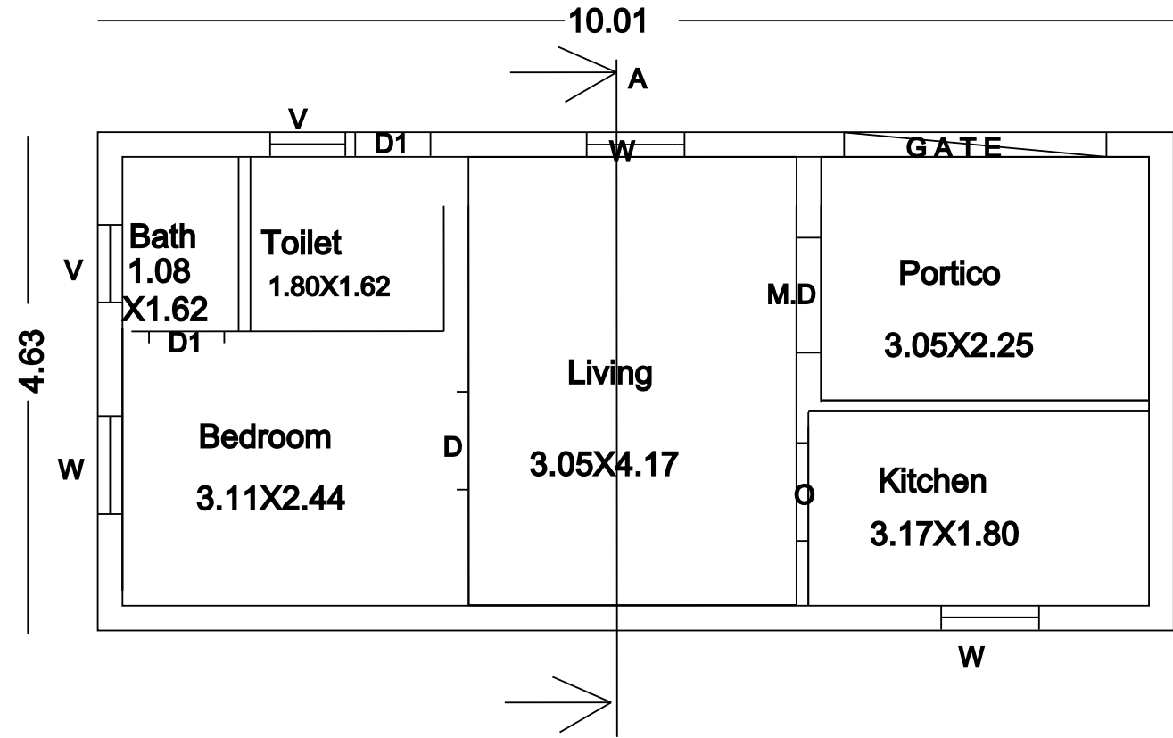
PRO. PLAN
