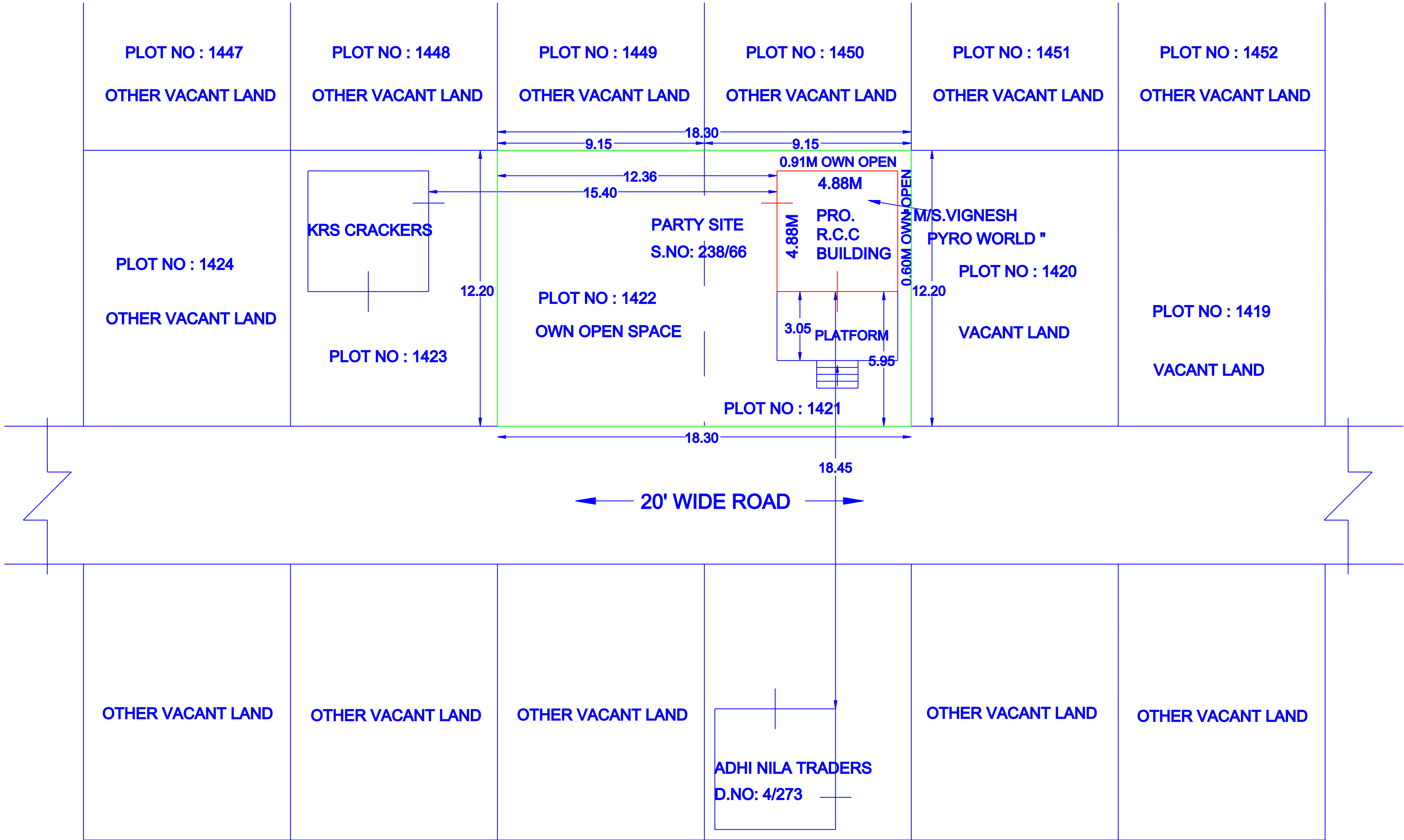
SITE PLAN SCALE - 1 : 2 M
