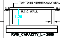
R.W.H. SECTION
