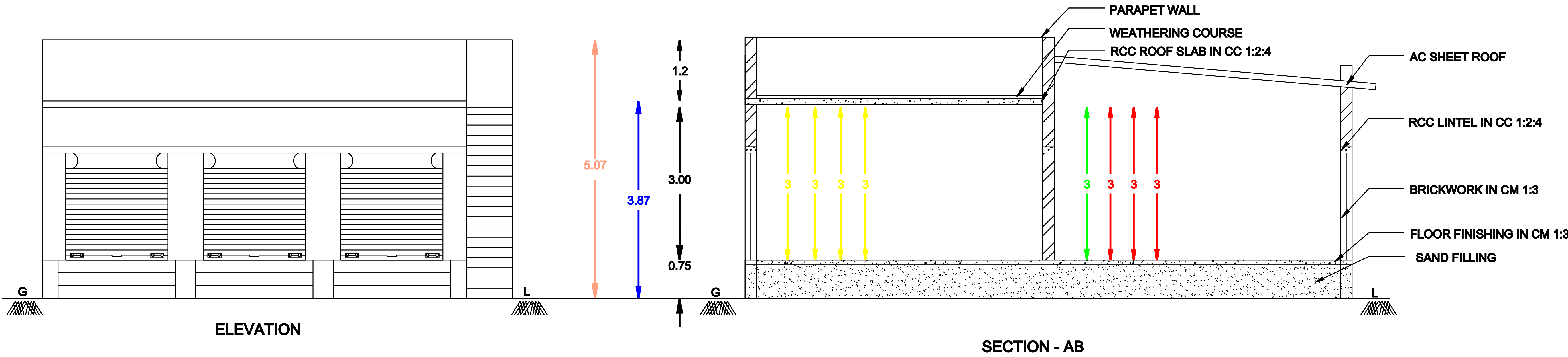
SECTION - AB
