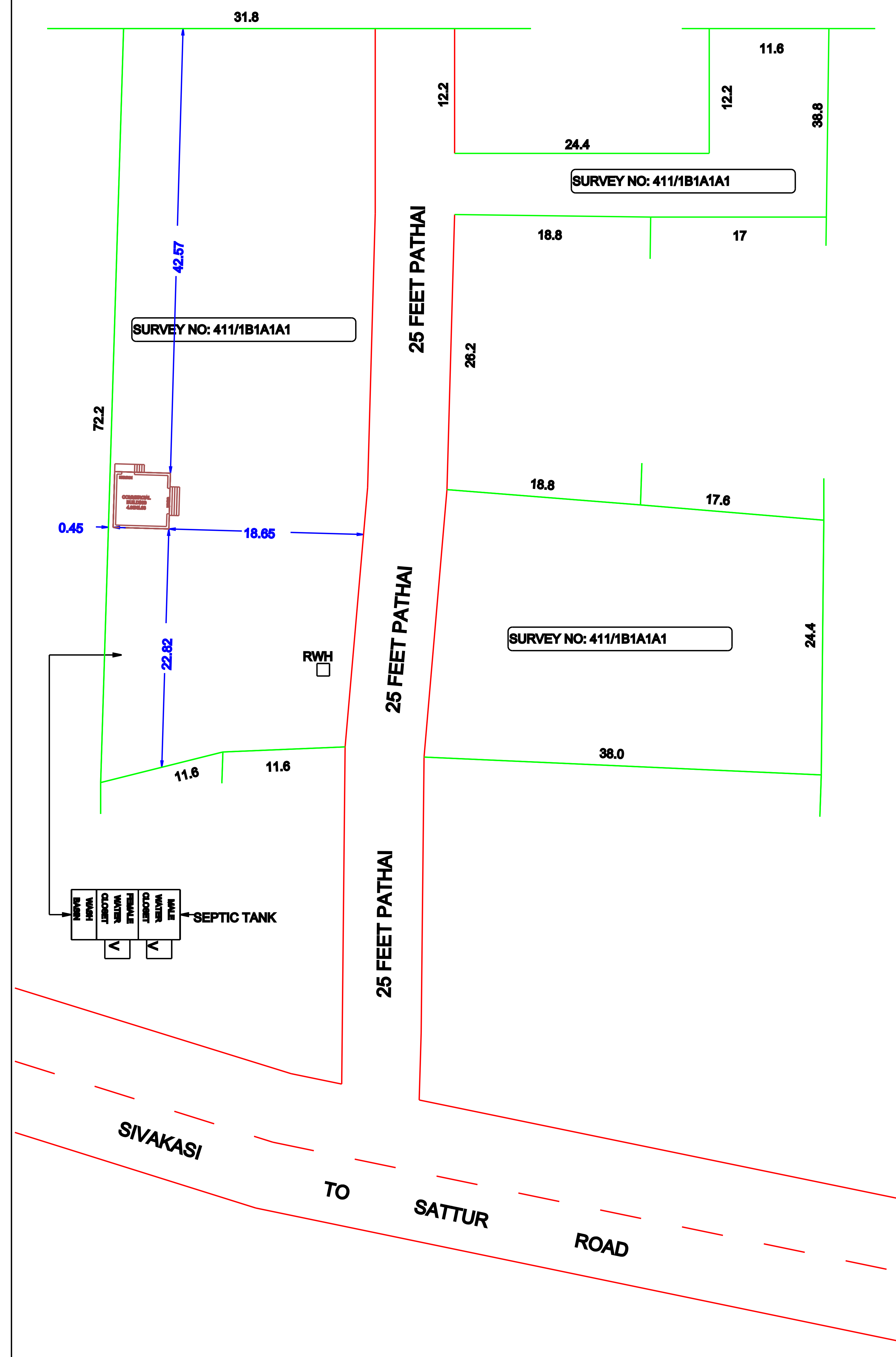
SITE PLAN SCALE 1:400
