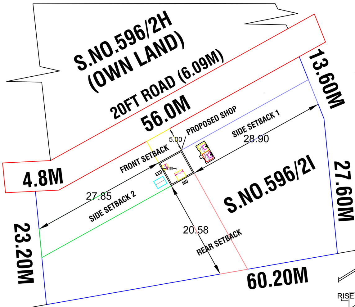
SITE CUM PLAN
