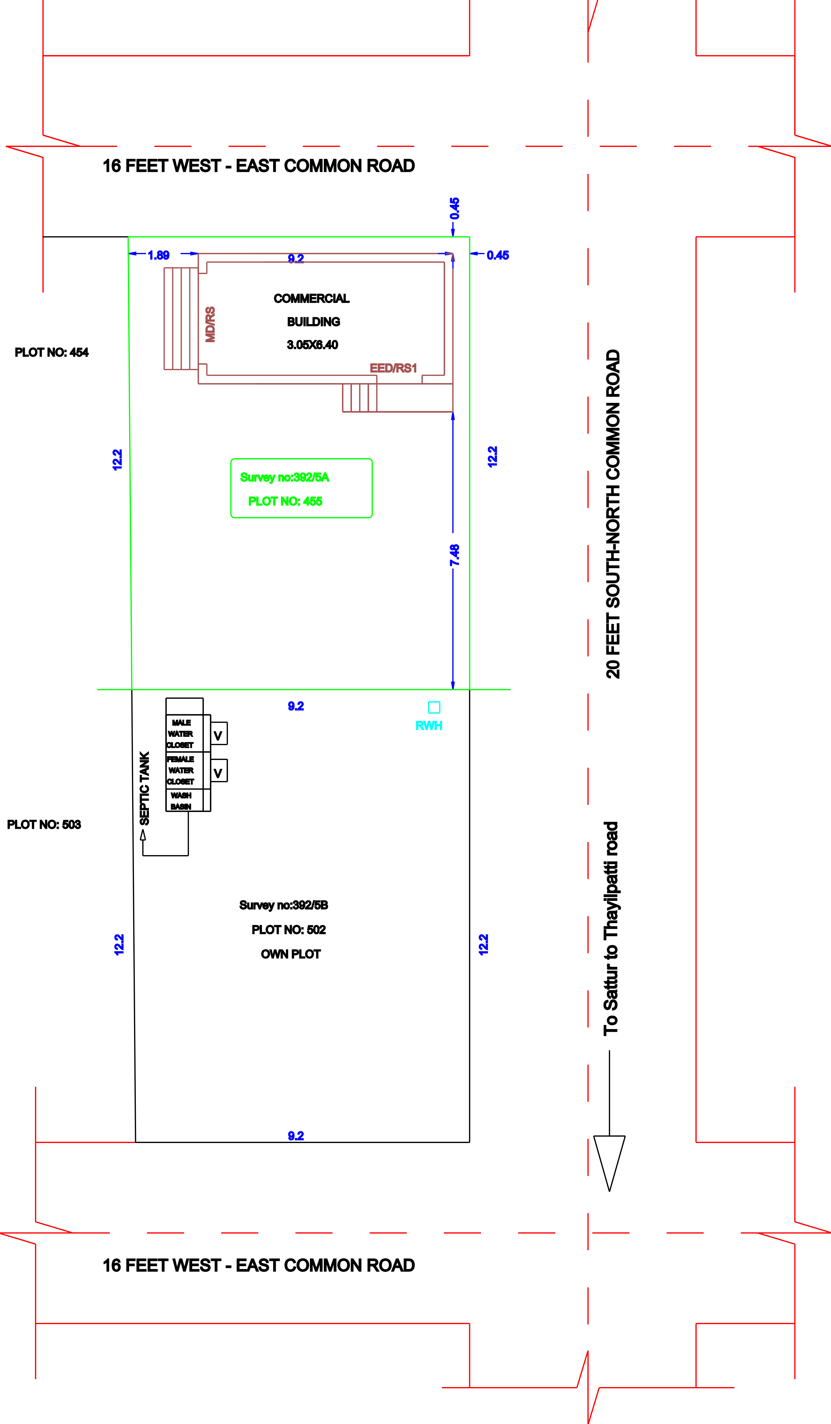
SITE PLAN 1:100
