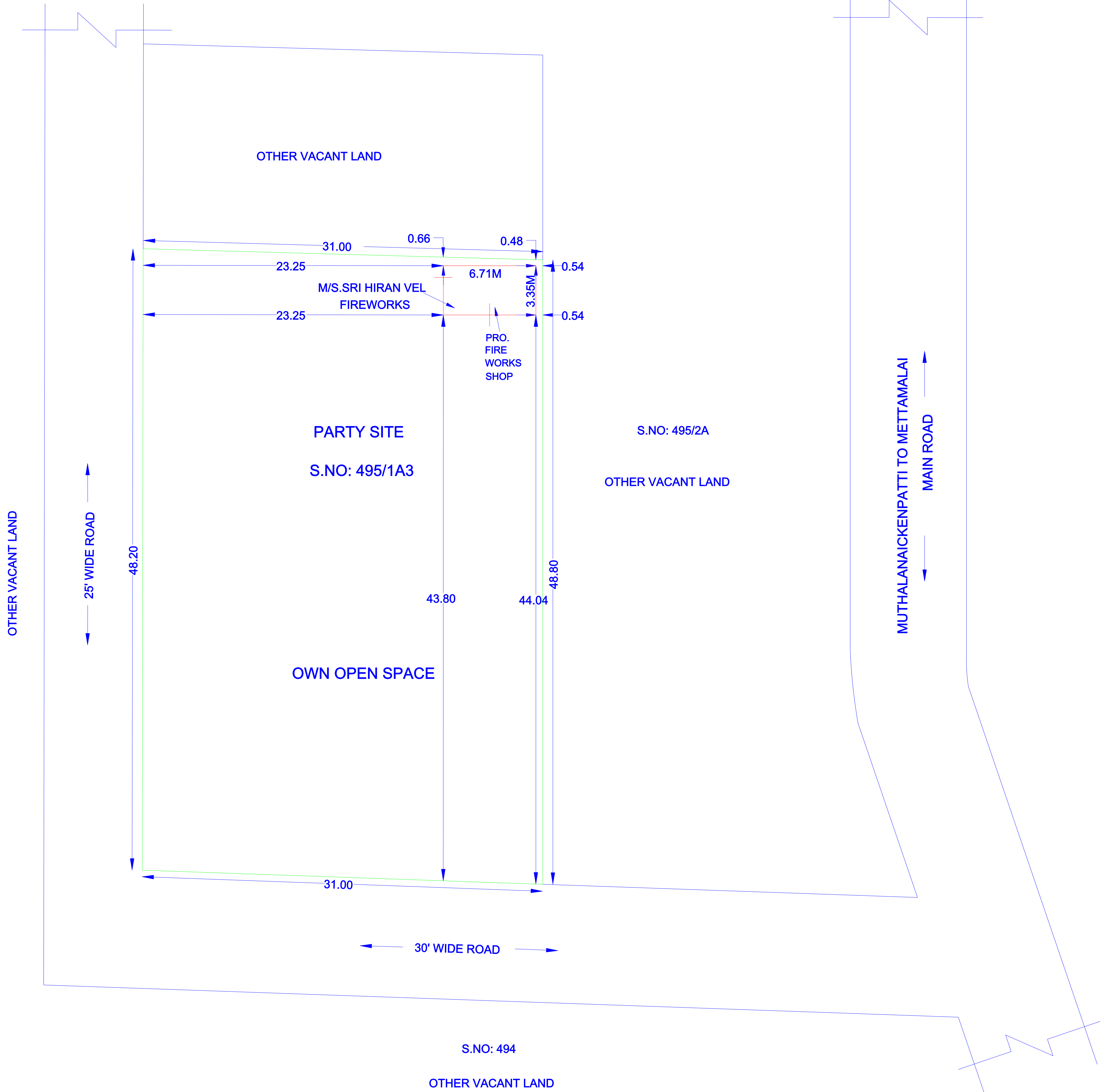
SITE PLAN SCALE - 1 : 3 M
