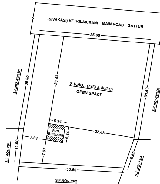
SITE PLAN (SCALE - 1:400)
