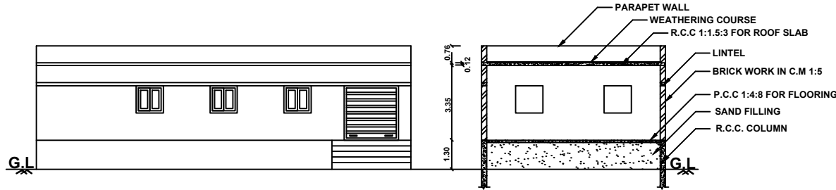
ELEVATION
