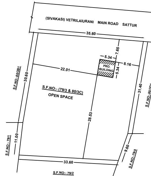
SITE PLAN (SCALE - 1:400)
