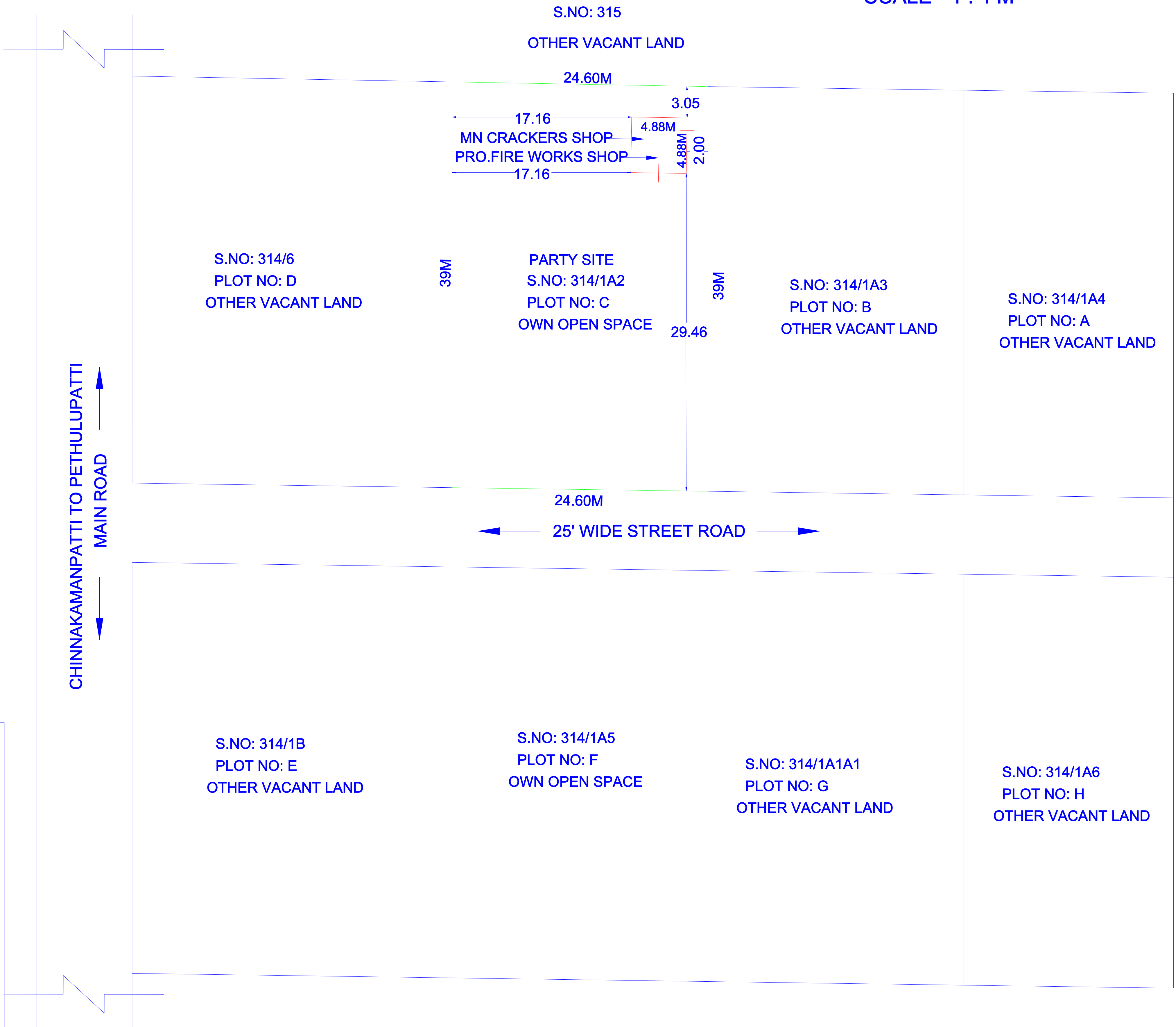
SITE PLAN SCALE - 1 : 4 M
