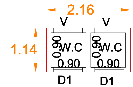
TOILET PLAN
