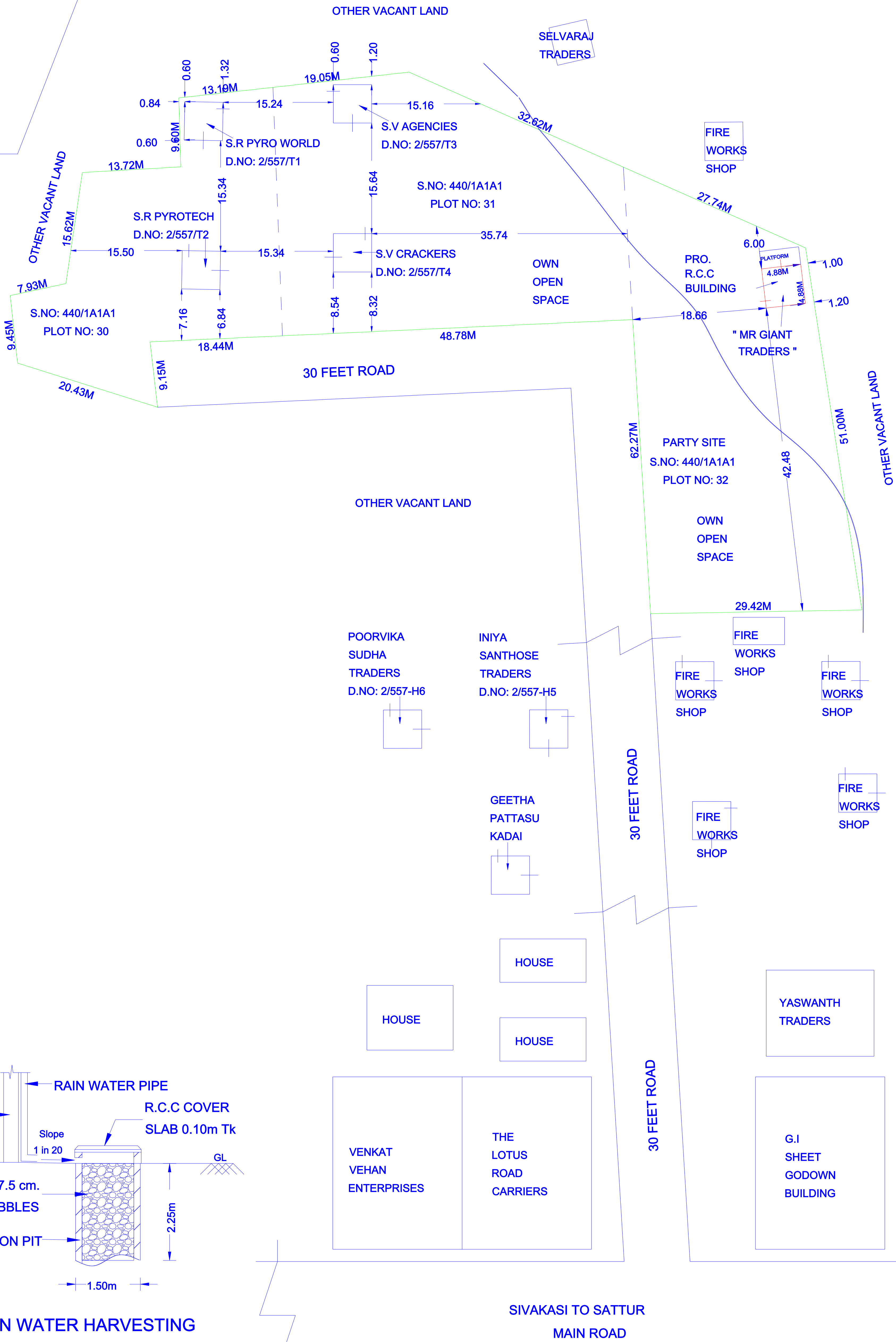
SITE PLAN SCALE - 1 : 6 M
