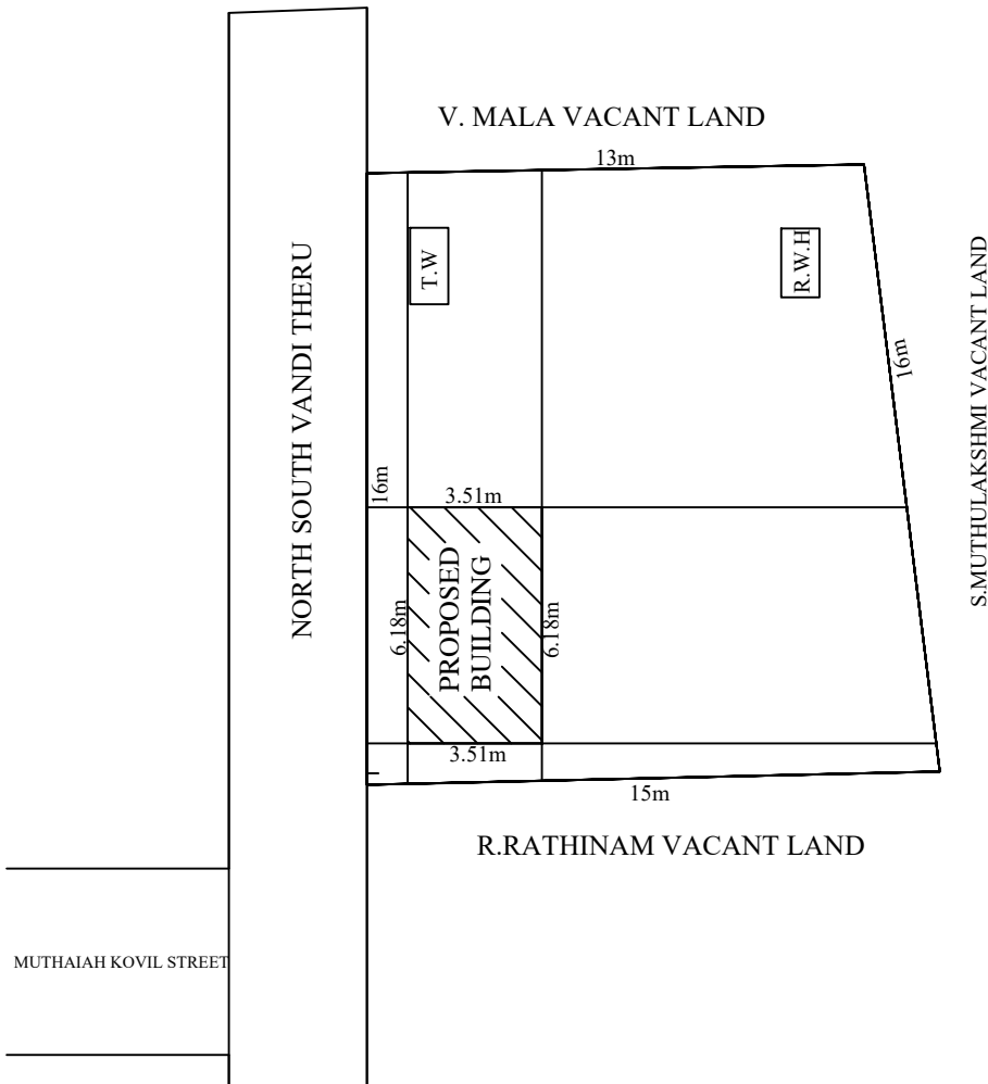
SITE PLAN 1:100
