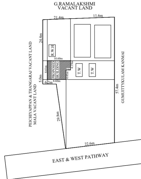
SITE PLAN 1:300
