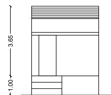
ELEVATION
