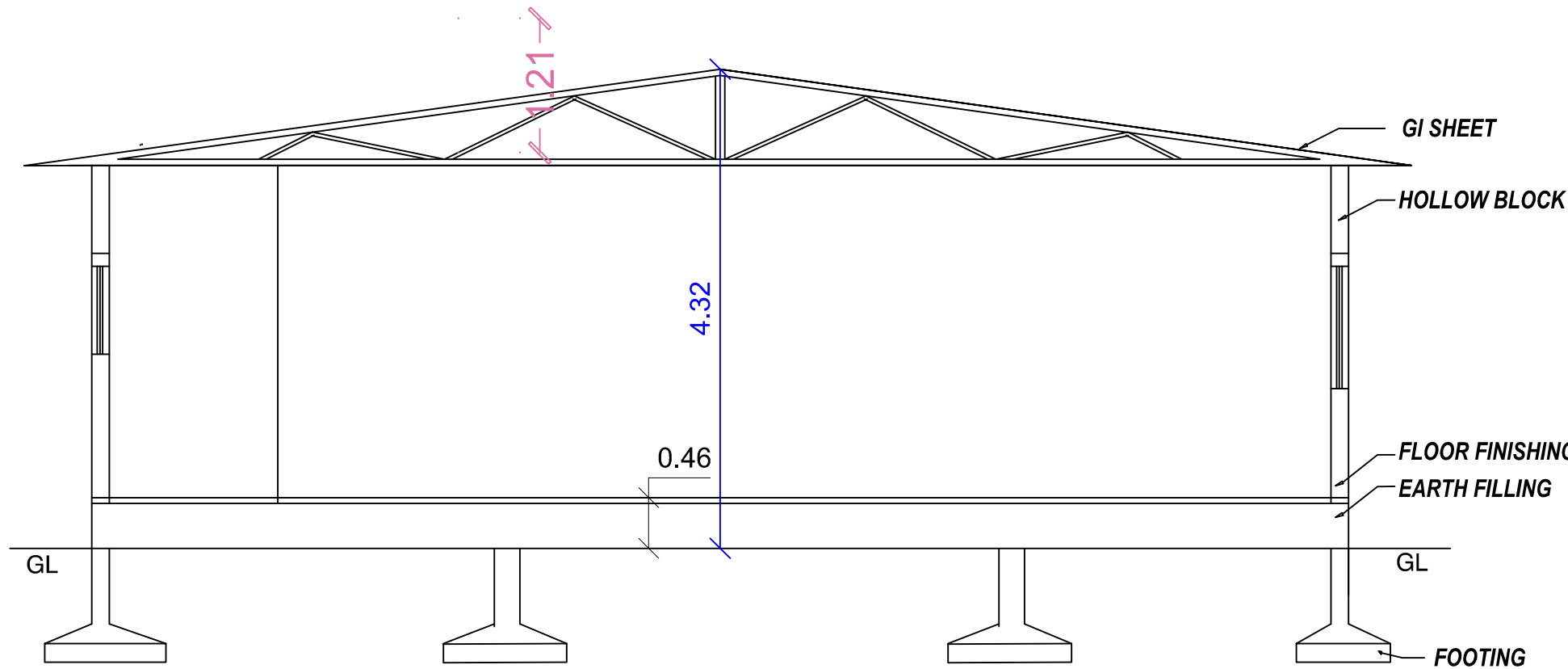
SECTION A-A1
