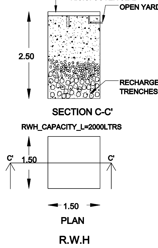
PLAN R.W.H
