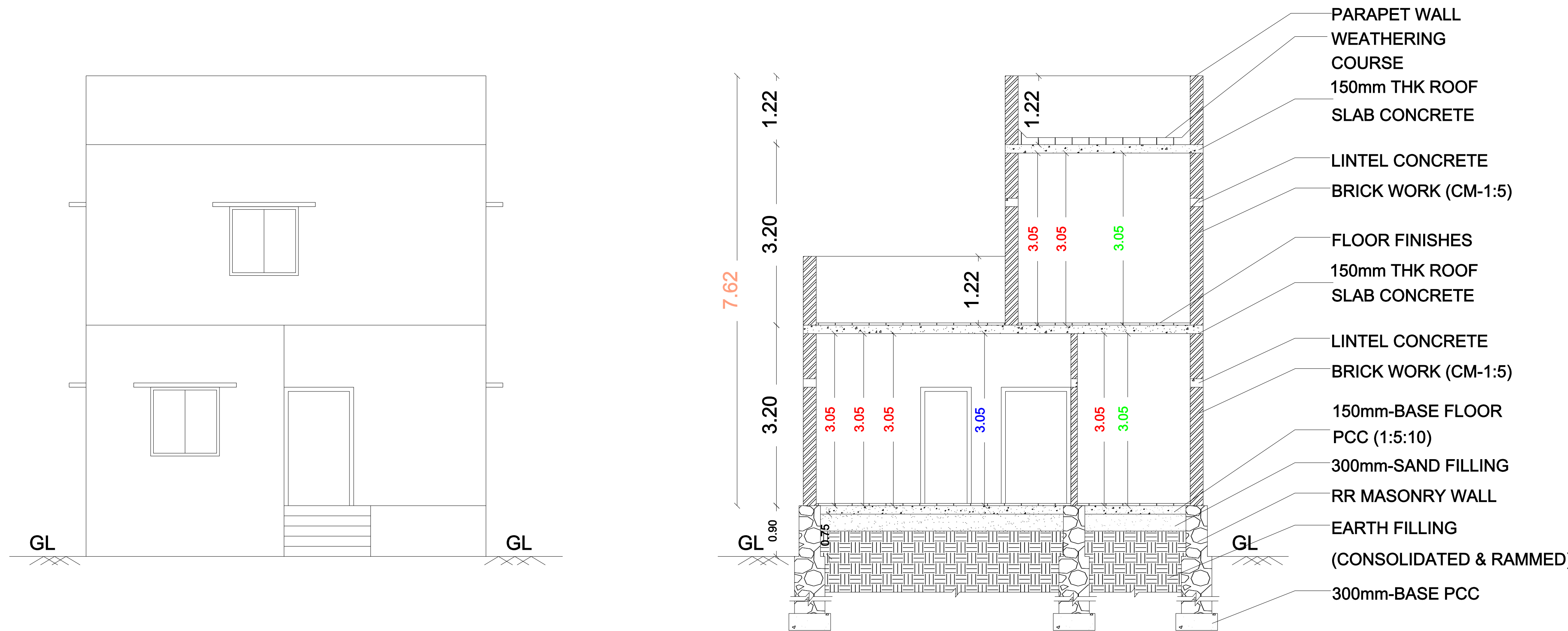
SECTION A-A
