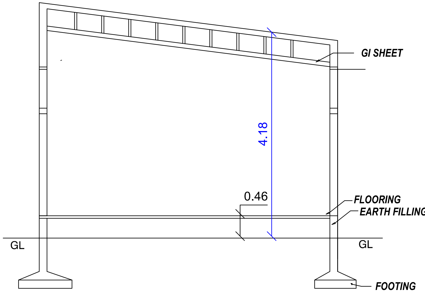
SECTION A-A1
