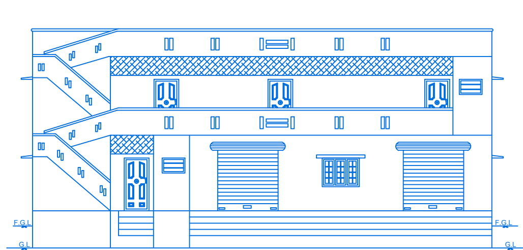
ELEVATION
