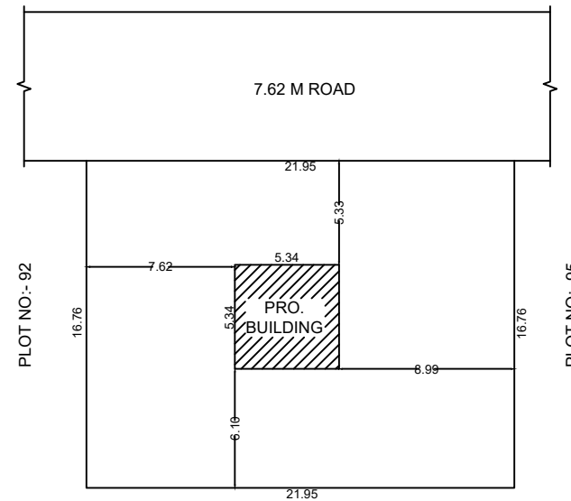
PLOT NO:- 139 & 140
