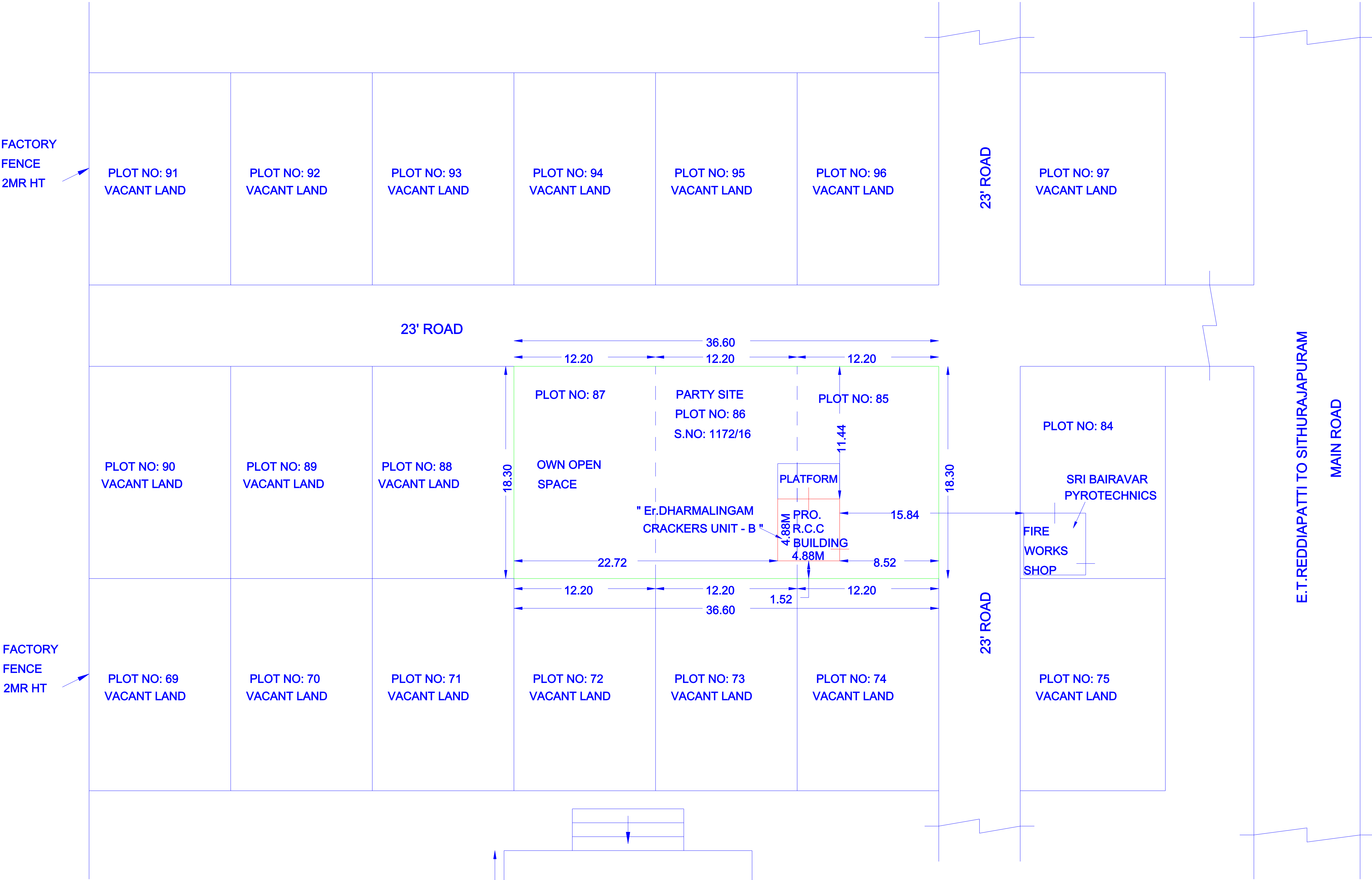
SITE PLAN SCALE - 1 : 4 M
