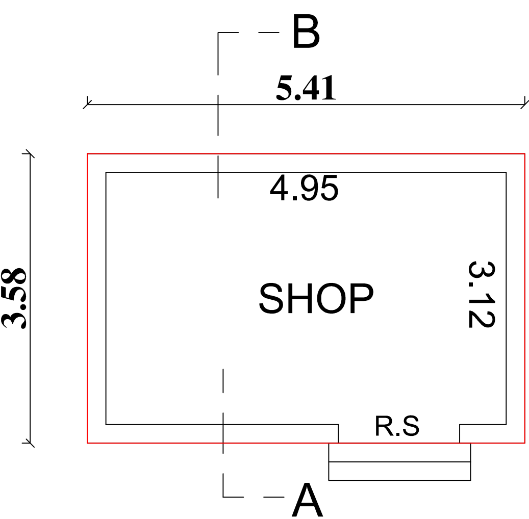
PLAN G.F
