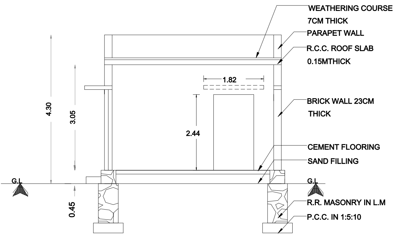
SECTION - AB
