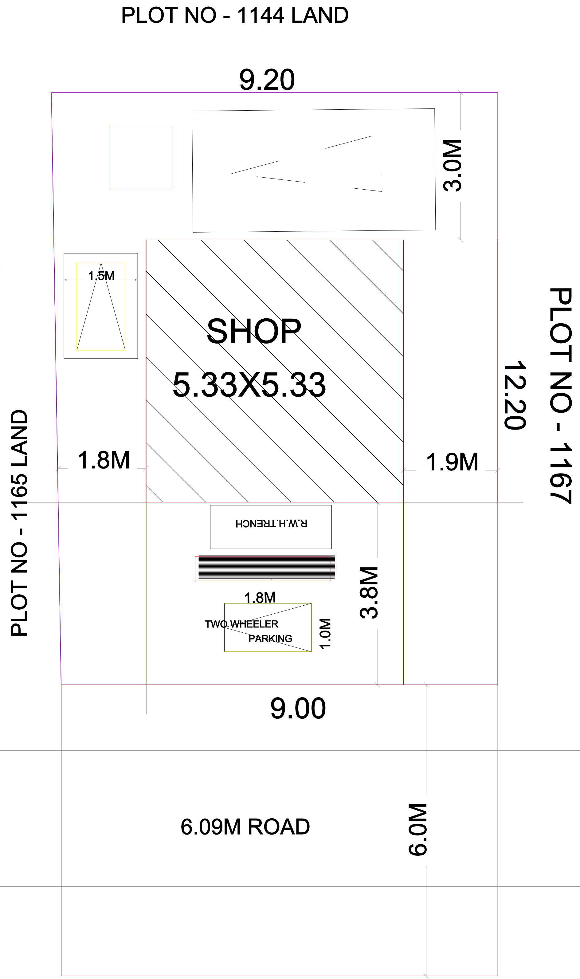
SITE PLAN - 1:100
